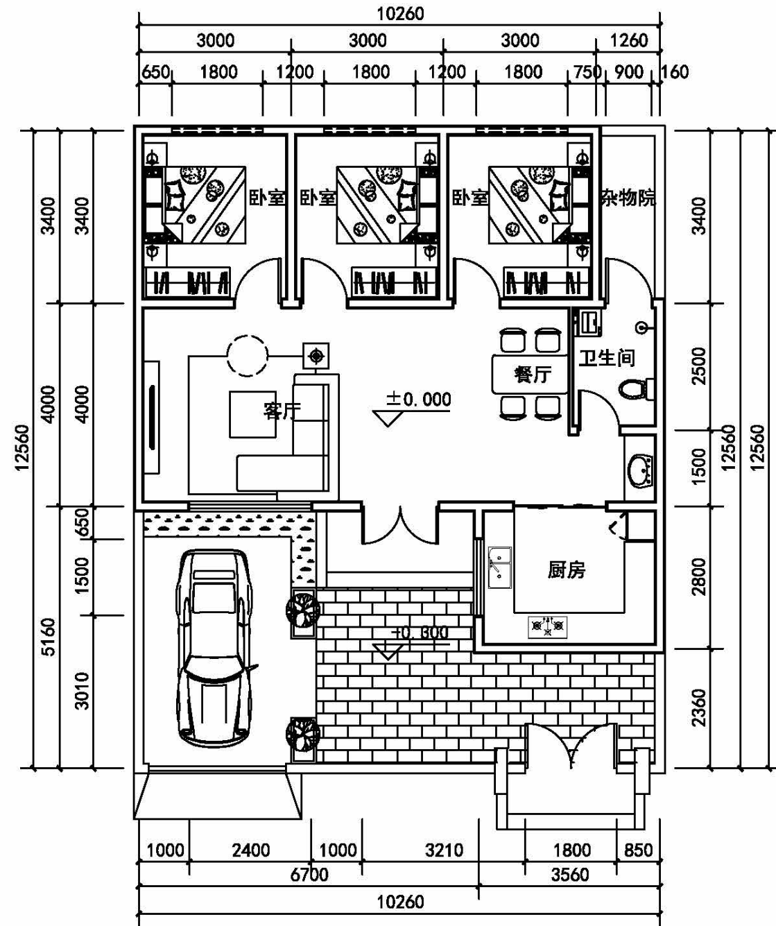
一层平面图 1:100
